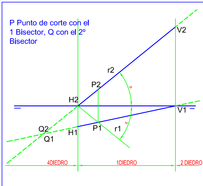
PARTES VISIBLES Y CORTES CON LOS BISECTORES
