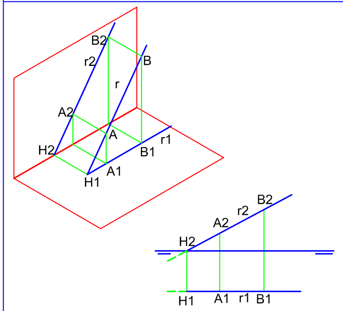
RECTA FRONTAL (PARALELA AL PLANO VERTICAL)
