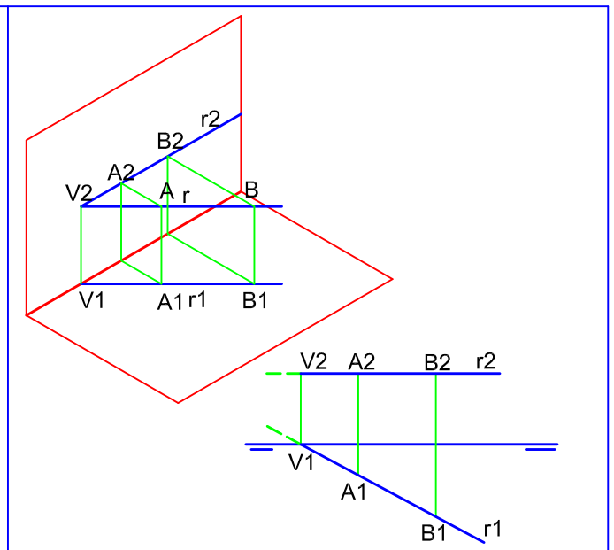
RECTA HORIZONTAL (PARALELA AL PLANO HORIZONTAL)
