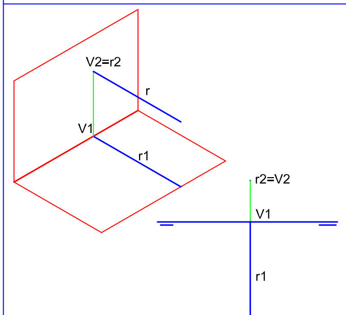
RECTA DE PUNTA (PERPENDICULAR AL PLANO VERTICAL)
