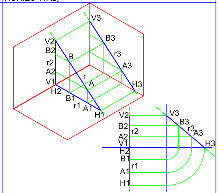
RECTA DE PERFIL (PARALELA AL PLANO DE PERFIL)
